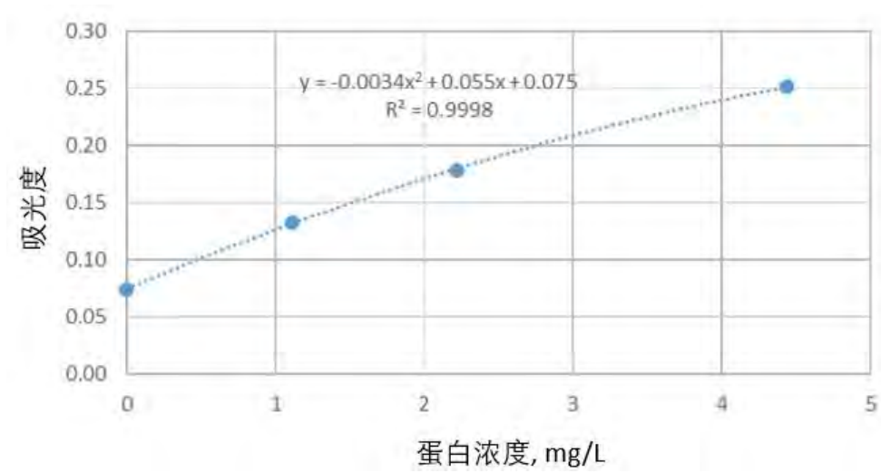
图 A.1 蛋白含量测定的标准曲线示意图
