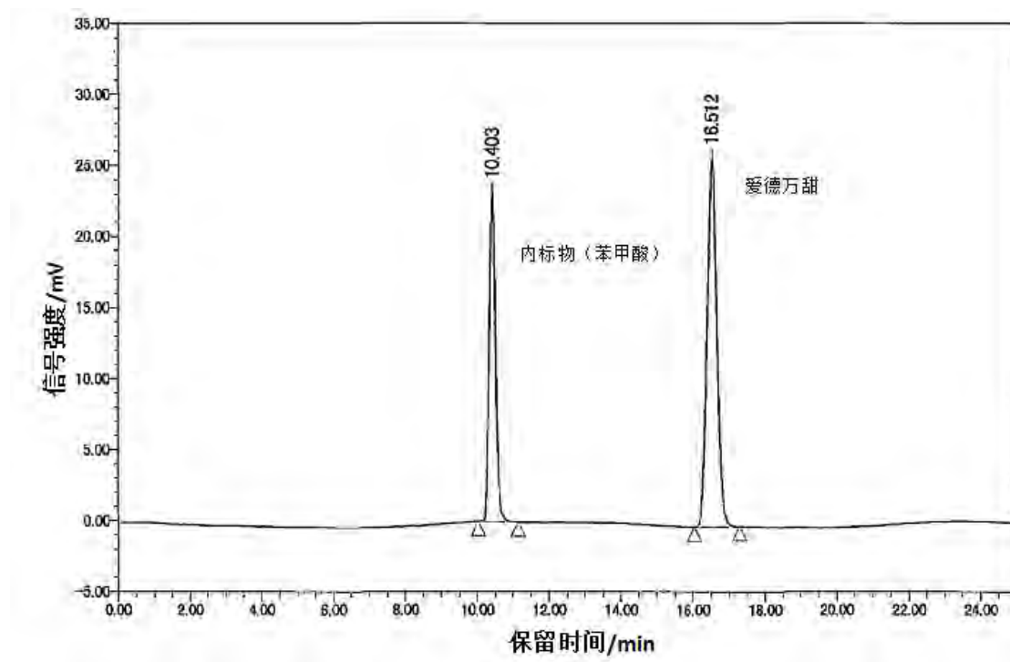
图 B.1 爱德万甜典型液相色谱图
