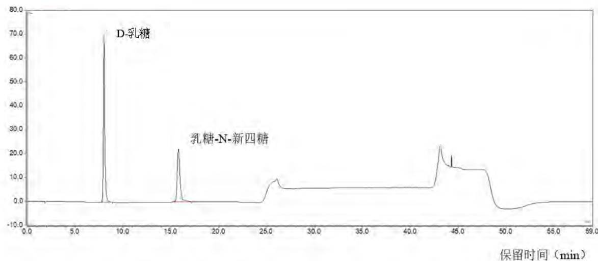
图 B.3 浓度为 0.01 mg/mL 的 D-乳糖和乳糖- N -新四糖对照品溶液的参考色谱图
